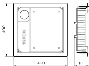
BBP500 LED180 PSU & PSD
